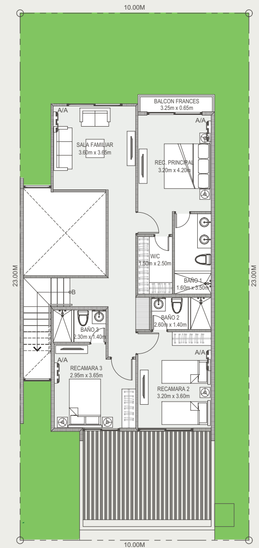
Planta Alta
